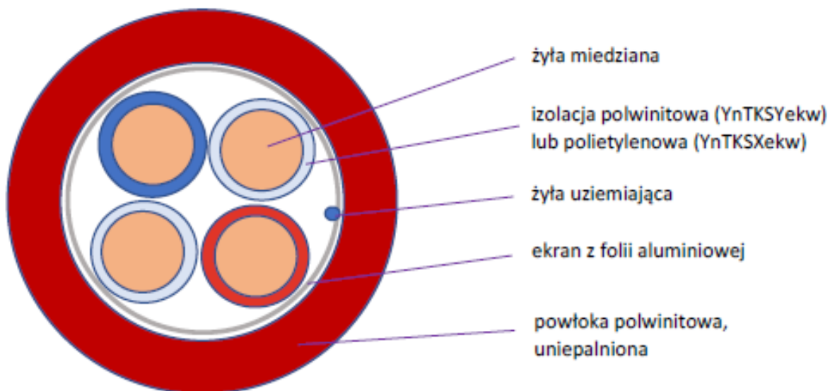
Ryc. 2. Przekrój kabla YnTKSYekw/YnTKSXekw Źródło: Materiały producenta.
