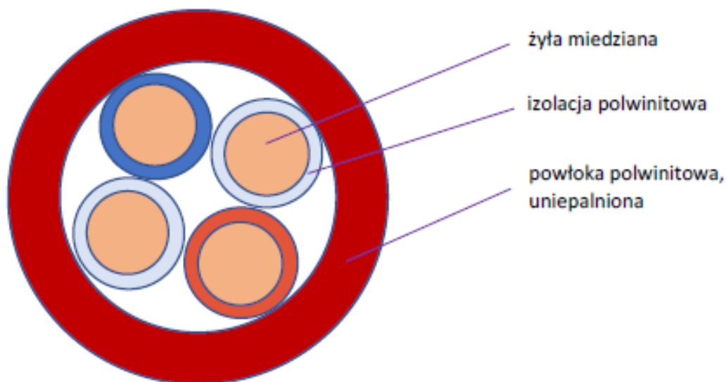
Ryc. 1. Przekrój kabla YnTKSY Źródło: Materiały producenta.
